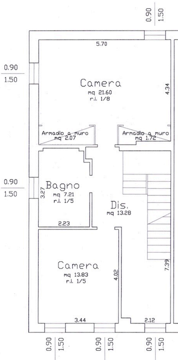
Piano Primo H=2.72
